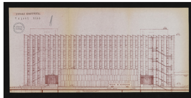
Elévation de la façade antérieure nord du projet définitif, s.d., ca. 1978. (Archives départementales de la Côte-d'Or, Dijon, 32 J 82) Phot. Petot Frédéric, Autr. Roger Martin Barade IVR26_20142100766NUC2A
