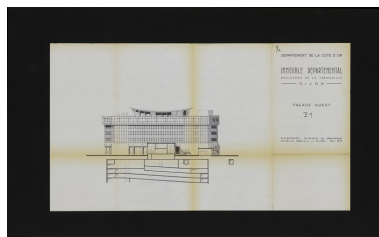
Premier projet : élévation de la façade postérieure ouest et coupe des niveaux en sous-sol, mai 1975. (Archives départementales de la Côte-d'Or, Dijon, 32 J 49) Phot. Petot Frédéric, Autr. Roger Martin Barade IVR26_20142100696NUC2A
