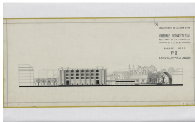
Deuxième projet : élévation de la façade antérieure nord, septembre 1975. (Archives départementales de la Côte-d'Or, Dijon, 32 J 462) Phot. Petot Frédéric, Autr. Roger Martin Barade IVR26_20142100811NUC2A
