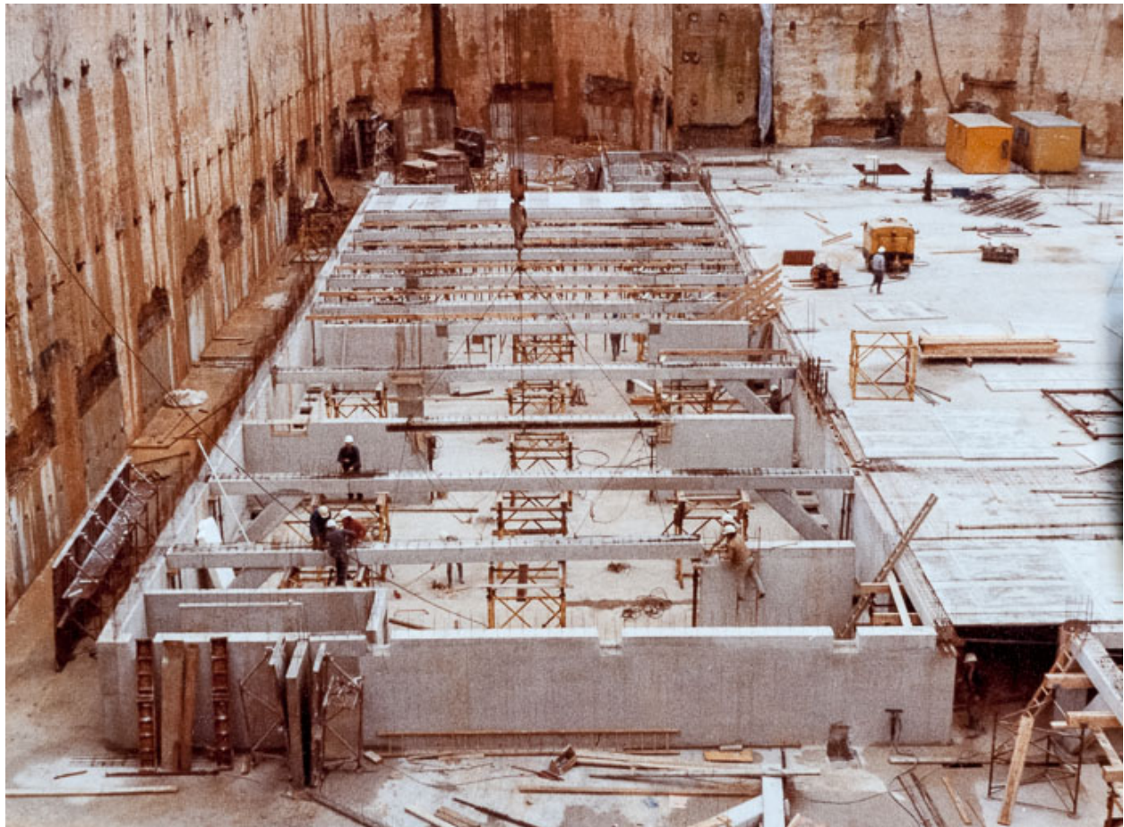
Vue du chantier en février 1978 : vue d'ensemble de la travée T1 du cinquième niveau du sous-sol et mise en place d'une poutre. Photographie ancienne. (Archives départementales de la Côte-d'Or, Dijon, 32 J 57)
