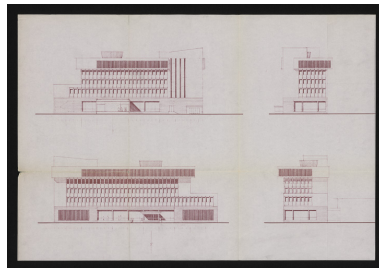
Variante du premier projet : élévations des façades antérieure, postérieure et latérale, ca. 1974-1975. (Archives départementales de la Côte-d'Or, Dijon, 32 J 49) Phot. Petot Frédéric, Autr. Roger Martin Barade IVR26_20142100691NUC2A
