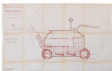
Plan du premier niveau du sous-sol, juin 1976. (Archives départementales de la Côte-d'Or, Dijon, 32 J 84) Phot. Pierre-Marie Barbe-Richaud, Autr. Roger Martin Barade
