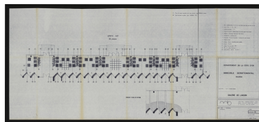
Plan de la galerie de liaison au rez-de-chaussée avec répartition des matériaux et du mobilier, 15 février 1979. (Archives départementales de la Côte-d'Or, Dijon, 32 J 106) Phot. Petot Frédéric, Autr. Michel (architecte d'intérieur) Boyer IVR26_20142100794NUC2A
