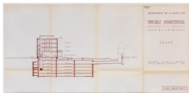
Coupe longitudinale, projet définitif, avril 1976. (Archives départementales de la Côte-d'Or, Dijon, 32 J 84) Phot. Pierre-Marie Barbe-Richaud, Autr. Roger Martin Barade IVR26_20142100603NUC2A
