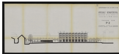
Deuxième projet : élévation de la façade postérieure sud, septembre 1975. (Archives départementales de la Côte-d'Or, Dijon, 32 J 50) Phot. Petot Frédéric, Autr. Roger Martin Barade IVR26_20142100743NUC2A
