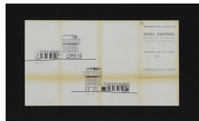
Premier projet : élévations des façades latérales sud et nord, mai 1975. (Archives départementales de la Côte-d'Or, Dijon, 32 J 49) Phot. Petot Frédéric, Autr. Roger Martin Barade IVR26_20142100697NUC2A
