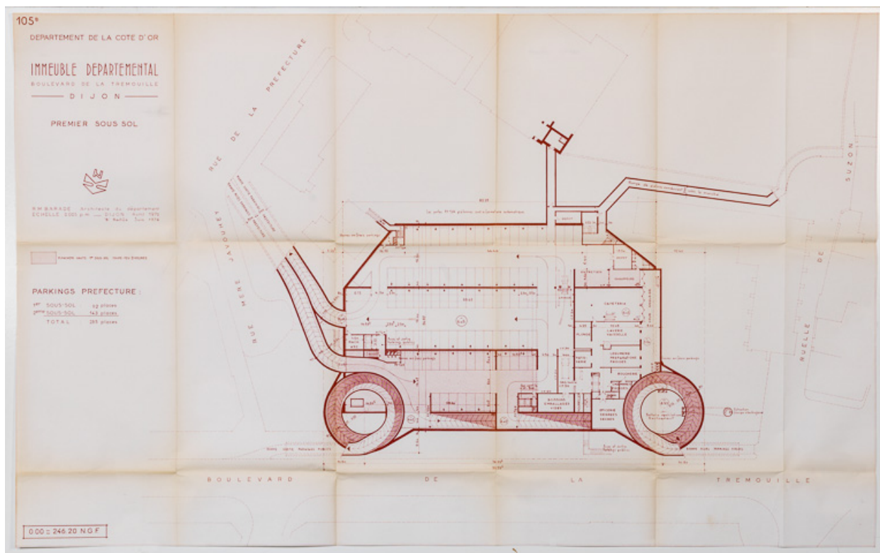
Plan du premier niveau du sous-sol, juin 1976. (Archives départementales de la Côte-d'Or, Dijon, 32 J 84)
