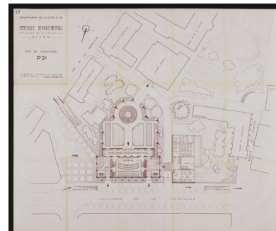
Deuxième projet : plan du rez-de-chaussée et des jardins, novembre 1975. (Archives départementales de la Côte-d'Or, Dijon, 32 J 50) Phot. Petot Frédéric, Autr. Roger Martin Barade IVR26_20142100746NUC2A
