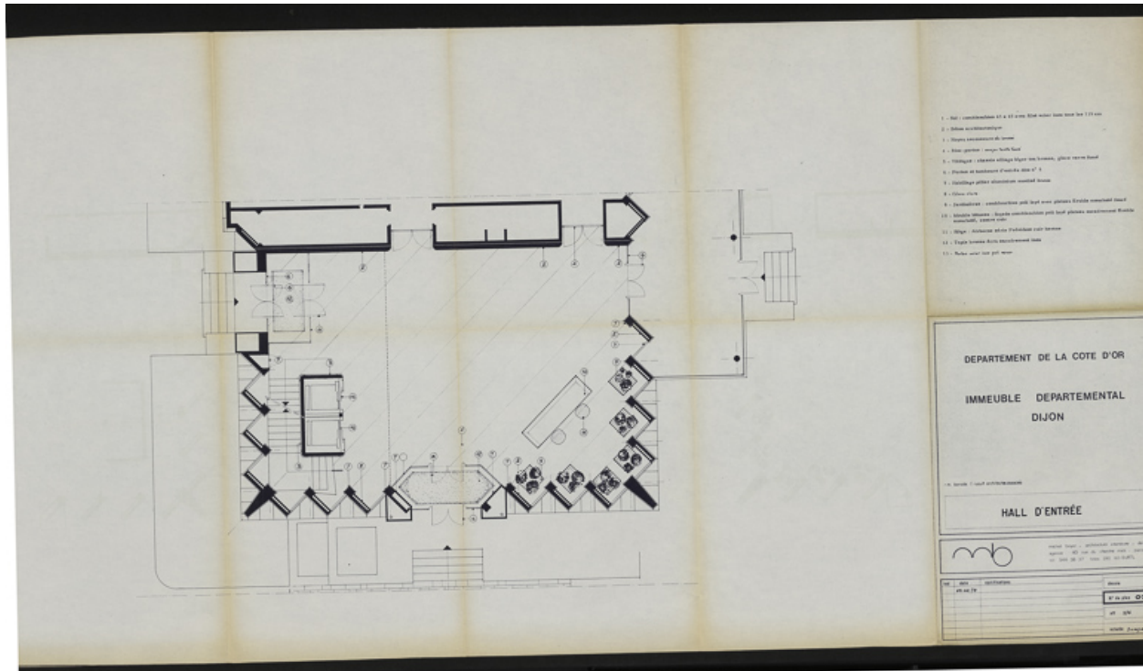
Plan du hall d'entrée au rez-de-chaussée avec répartition des matériaux et du mobilier, 15 février 1979. (Archives départementales de la Côte-d'Or, Dijon, 32 J 106)
