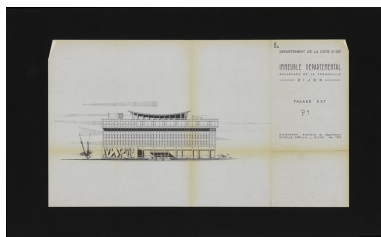
Premier projet : élévation de la façade antérieure est, mai 1975. (Archives départementales de la Côte-d'Or, Dijon, 32 J 49) Phot. Petot Frédéric, Autr. Roger Martin Barade IVR26_20142100695NUC2A
