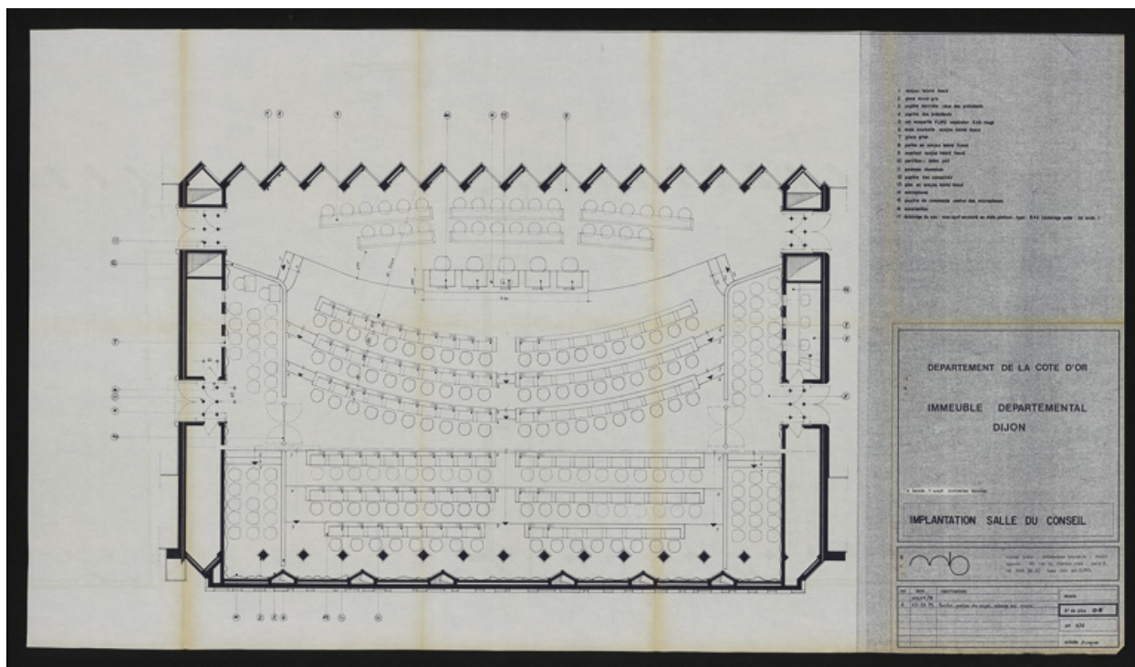
Plan de la salle des assemblée au rez-de-chaussée avec implantation des matériaux et du mobilier, 15 février 1979. (Archives départementales de la Côte-d'Or, Dijon, 32 J 106)
