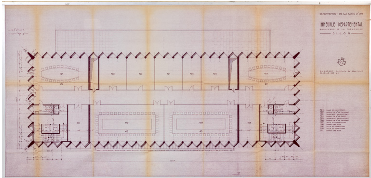
Plan du premier étage, non daté, ca. 1976. (Archives départementales de la Côte-d'Or, Dijon, 32 J 84)
