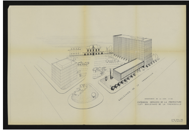
Projet d'extension des services de la préfecture (non réalisé), élévation perspective, avril 1962. (Archives départementales de la Côte-d'Or, Dijon, 32 J 48) Phot. Petot Frédéric, Autr. Roger Martin Barade IVR26_20142100633NUC2A
