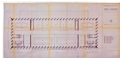
Plan du premier étage, non daté, ca. 1976. (Archives départementales de la Côte-d'Or, Dijon, 32 J 84) Phot. Pierre-Marie Barbe-Richaud, Autr. Roger Martin Barade IVR26_20142100604NUC2A
