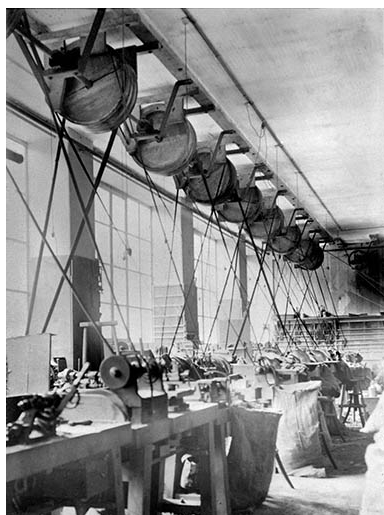
Ground Floor. Ebauchage [Rez-de-chaussée. Ebauchage en 1910]. Phot. Jérôme Mongreville IVR43_19923900137X
