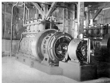
Engine, Generator & Exciter [Moteur, générateur et excitatrice en 1910]. Phot. Jérôme Mongreville IVR43_19923900128X
