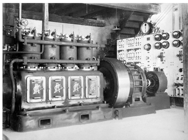
Generating set & Switchboard [Ensemble générateur et tableau de contrôle en 1910]. Phot. Jérôme Mongreville IVR43_19923900129X
