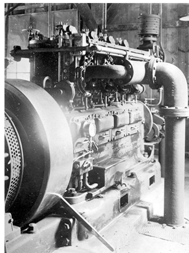
Engine, showing starting handles [Moteur, montrant les manettes de démarrage en 1910]. Phot. Jérôme Mongreville IVR43_19923900130X
