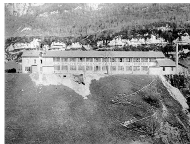
St Blaise Factory. Side facing River [Usine de Saint-Blaise. Façade du côté de la rivière en 1910]. Phot. Jérôme Mongreville IVR43_19923900127X
