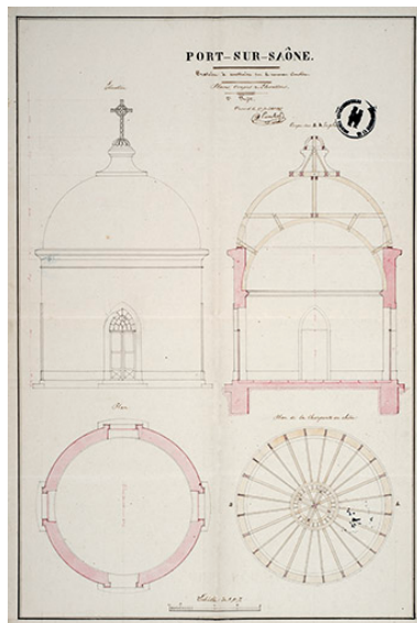
Oratoire à construire au nouveau cimetière : plan, coupe et élévation (2ème projet). Phot. Jérôme Mongreville, Autr. Jean-Baptiste Pambet, Autr. Servas IVR43_20177001149NUC4A
