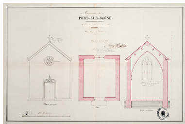
Oratoire à construire au nouveau cimetière : plan, coupe et élévation (1er projet). Phot. Jérôme Mongreville, Autr. Jean-Baptiste Pambet, Autr. Servas IVR43_20177001148NUC4A
