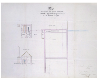
Plan dressé à l'appui d'une demande en autorisation d'appareils à vapeur établis dans le moulin à ciment de M. Lesmann à Roppe. Phot. Jérôme Mongreville IVR43_20019000059VA
