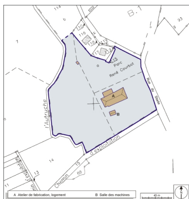
Plan-masse et de situation. Extrait du plan cadastral, 2001, section ZB, 1:2000 agrandi à 1:1500. Dess. André Céréza IVR43_20039000056NUDA
