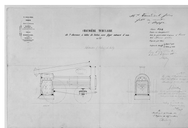
Chaudière tubulaire de 9 chevaux, à tubes de laiton, avec foyer entouré d'eau (F. Calla fils, Paris). Phot. Jérôme Mongreville, Autr. Félix Schneider IVR43_20019000024V
