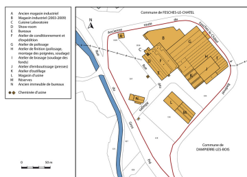
Plan-masse et de situation. Dess. Mathias Papigny IVR43_20132502574NUDA
