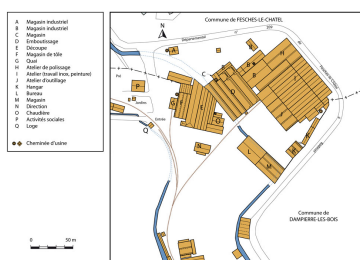
Plan-masse de l'usine en 1977. D'après un extrait du plan cadastral. Dess. Mathias Papigny IVR43_20142500610NUDA
