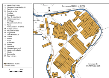
Plan-masse de l'usine en 1939. D'après le plan général de la Casserie, 1939. Dess. Mathias Papigny IVR43_20142500609NUDA
