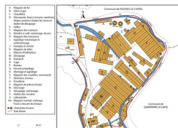
Plan-masse de l'usine en 1895. D'après le plan général de la Casserie, 1895. Dess. Mathias Papigny IVR43_20142500608NUDA
