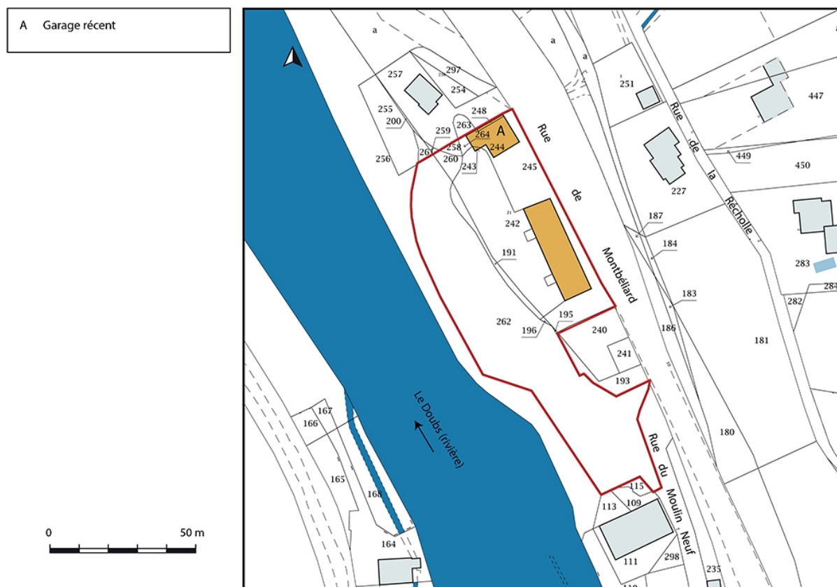
Plan-masse et de situation. Extrait du plan cadastral, 2019, section AB.
