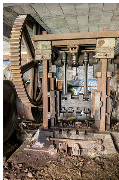
Presse à forger. Phot. Jérôme Mongreville IVR43_20152501245NUC4A
