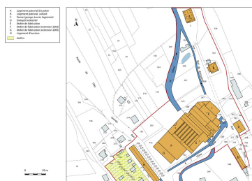
Plan-masse et de situation. Dess. Mathias Papigny IVR43_20132502641NUDA
