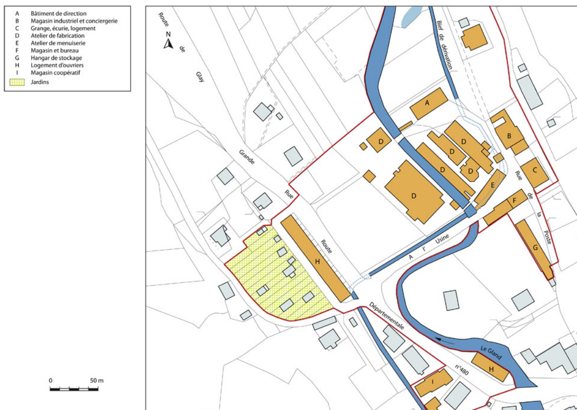
Plan-masse de l'usine vers 1980.
