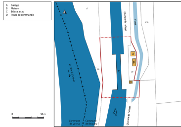
Plan masse et de situation. Dess. Bertrand Turina IVR43_20207000797NUDA
