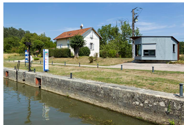
L'écluse, le poste de commande et la maison d'éclusier. Phot. Sonia Dourlot IVR43_20157000859NUC4A
