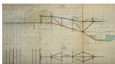
Exploitation militaire du Canal du Rhône au Rhin. Installation de transbordement au port des Près-de-Vaux, à Besançon. Projet définitif. Dessins du transbordeur [détail : plan et élévation], 1918. Phot. Yves Sancey, Autr. Bérard IVR43_20062500059NUCA
