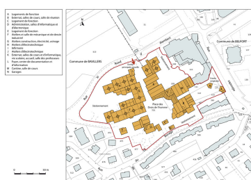
Plan-masse et de situation. Extrait du plan cadastral numérisé, section AD, échelle 1:1000. Dess. Mathias Papigny IVR43_20149000152NUDA
