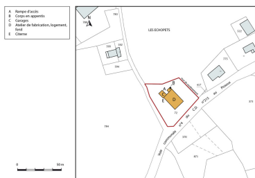
Plan-masse et de situation. Dess. Mathias Papigny IVR43_20162501551NUDA
