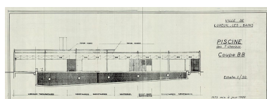
Coupe longitudinale de la piscine sur le bassin. IVR43_20267000067NUC4A
