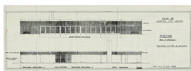
Élévations des faces nord- est (entrée) et nord-ouest. IVR43_20267000069NUC4A
