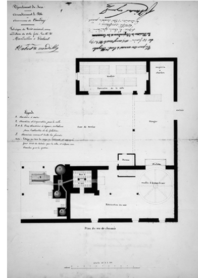
Fabrique de noir animal avec addition de colle forte par MM Mandrillon et Dubant. Plan du rez-de-chaussée.
