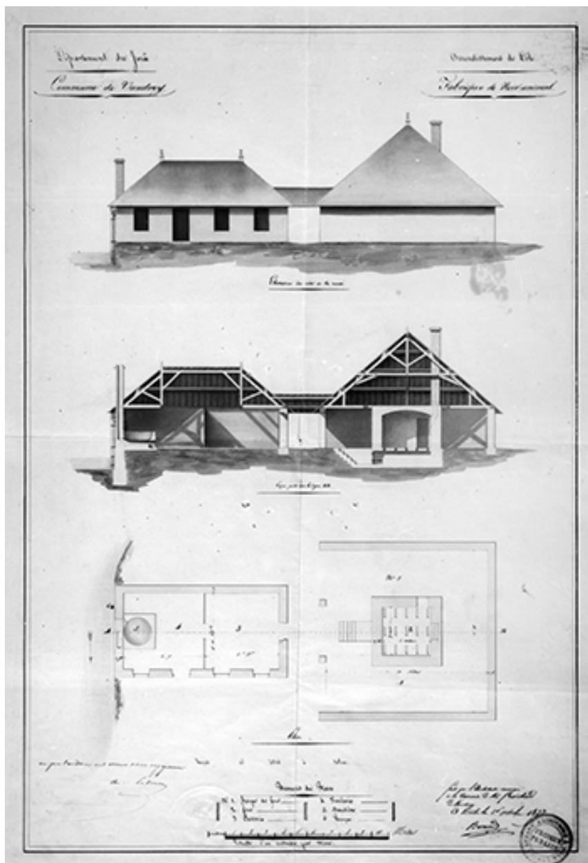
Fabrique de noir animal, plan, coupe et élévation.
