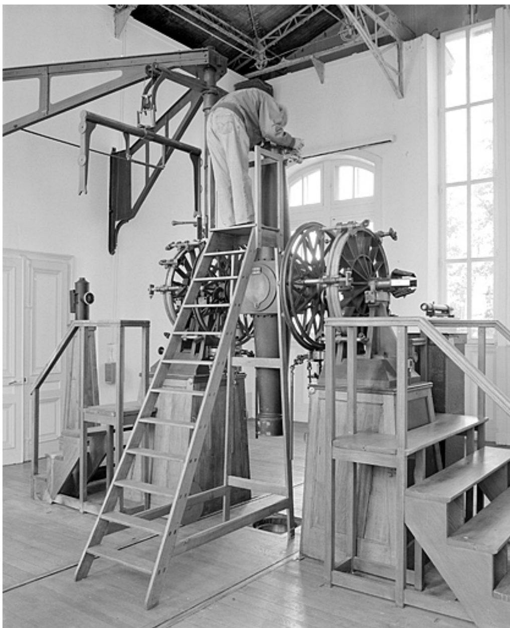
Utilisation de l'escabeau à marches, avec la lunette à la verticale pour les observations nadirales.
