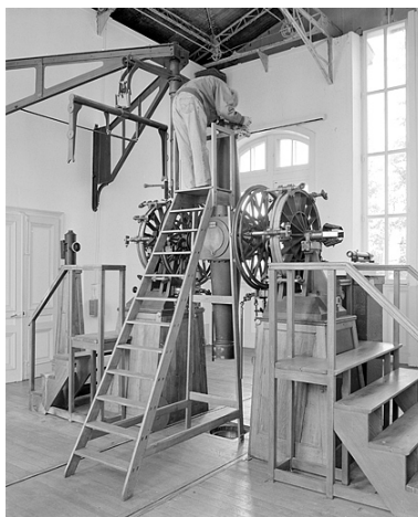
Utilisation de l'escabeau à marches, avec la lunette à la verticale pour les observations nadirales. Phot. Jérôme Mongreville IVR43_20042500033X
