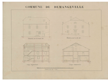
Plan de l'école : élévation et coupe. Phot. Philippe Mairot IVR43_20167000151NUC4A
