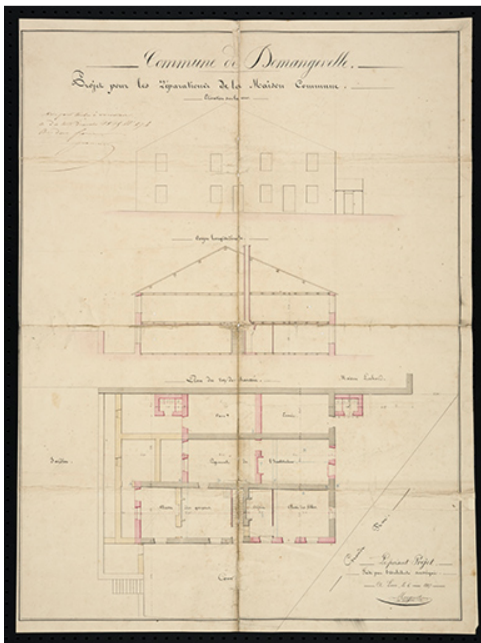
Plan : projet pour les réparations de la maison commune. (1835)
