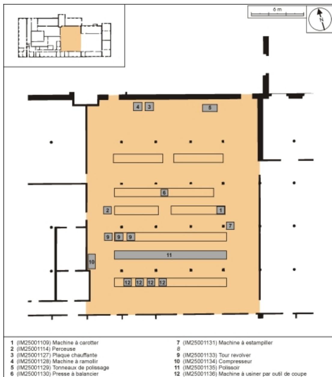
Plan de localisation des machines de la ligne de fabrication commune aux pipes en bruyère et aux pipes en merisier. Atelier principal.
