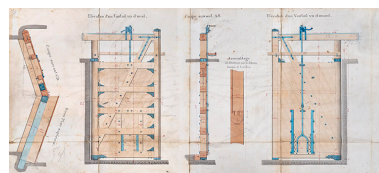
Achèvement de la dérivation de St-Albin (en aval du souterrain) - Portes d'écluse d'amont (1876). Phot. Jérôme Mongreville, Autr. Gustave Bouvaist IVR43_20207000077NUC4A
