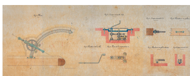
Achèvement de la dérivation de St-Albin (en aval du souterrain) - appareil de manœuvre des portes de l'écluse (1876). Phot. Jérôme Mongreville, Autr. Gustave Bouvaist IVR43_20207000074NUC4A
