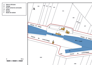
Plan-masse et de situation. Extrait du plan cadastral, 1876. Dess. Bertrand Turina IVR43_20197000169NUDA
