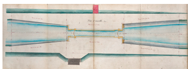
Achèvement de la dérivation de St-Albin (en aval du souterrain) - Ecluse à sas (1876). Phot. Jérôme Mongreville, Autr. Gustave Bouvaist IVR43_20207000078NUC4A
