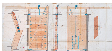
Achèvement de la dérivation de St-Albin (en aval du souterrain) - Portes d'écluse d'aval (1876). Phot. Jérôme Mongreville, Autr. Gustave Bouvaist IVR43_20207000076NUC4A
