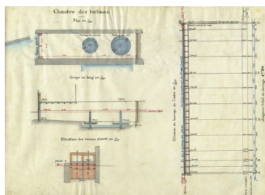
Commune de Morteau. Réglementation d'eau de l'usine des consorts Pertusier. Dessins de détail [... chambre des turbines], 5 juin 1897. Autr. Guiot-Guillain
