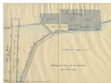
Commune de Morteau. Réglementation d'eau de l'usine des consorts Pertusier. Dessins de détail [... de l'usine et du barrage], 5 juin 1897. Autr. Guiot-Guillain IVR43_20182500038NUC4A
