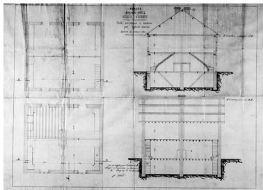
Forges de Franche-Comté. Mine d'Ougney. Plan d'un bâtiment à construire pour logements d'ouvriers [deux travées de la " Caserne "]. Phot. Yves Sancey IVR43_19883900280V
