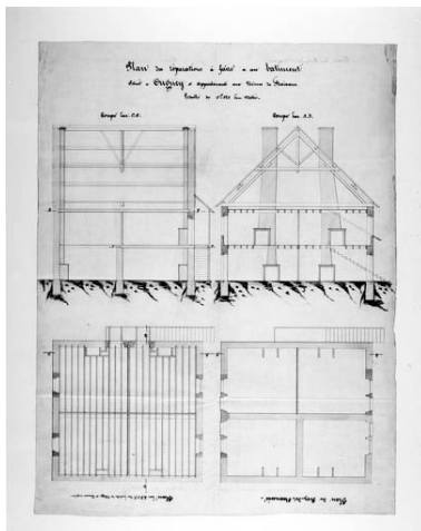
Plan des réparations à faire à un bâtiment situé à Ougney et appartenant aux usines de Fraisans (bâtiment non localisé). Phot. Yves Sancey IVR43_19883900278V
