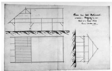
Plan d'un petit bâtiment à construire à Ougney pour servir d'écurie et de hangar à fourrage. Phot. Yves Sancey IVR43_19883900277V
