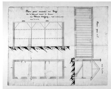
Plan pour remonter un étage sur le bâtiment servant de bureau aux mines d'Ougney. Phot. Yves Sancey IVR43_19883900276V
