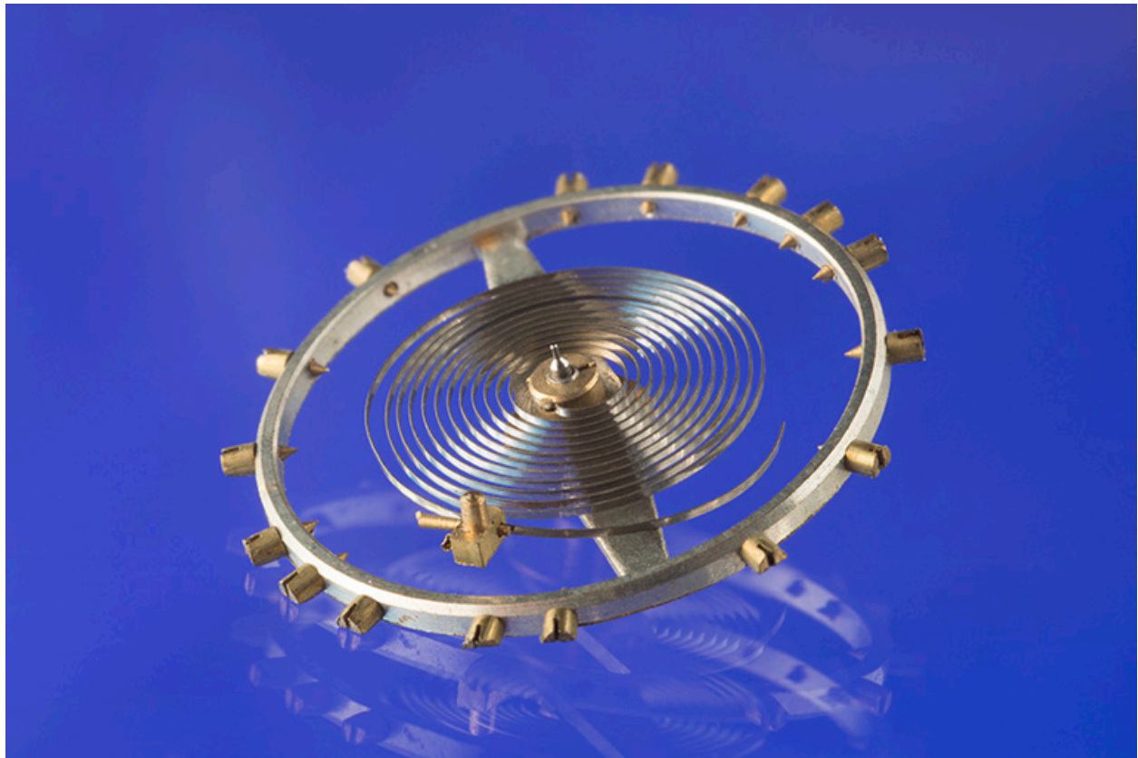
Le balancier-spiral, organe réglant de la montre.
