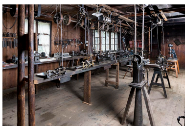
Atelier de fabricant d'outillage d'horlogerie, aux Gras. Phot. Sonia Dourlot IVR43_20172500036NUC4A
