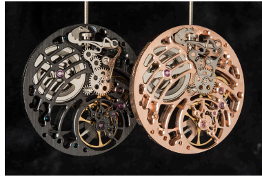
Mouvements de montre mécanique Arte de la société Berthet Horlogerie, Charmauvillers et Villers-le-Lac, 2018. Phot. Sonia Dourlot IVR43_20182501160NUC4A
