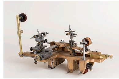
Machine à meuler et limer ("machine à passer les levées" pour la fabrication de l'échappement à cylindre), par Léon Girardin au Russey, 4e quart 19e siècle. Phot. Sonia Dourlot IVR43_20192500434NUC4A
