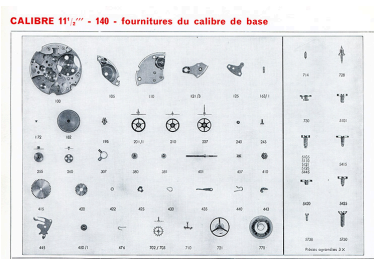
Calibre 11 1/2''' - 140 - fournitures du calibre de base [FE 140], 1973. IVR43_20162500135NUC2A
