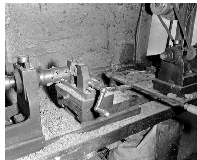
Mèche et chariot mobile. Phot. Jérôme Mongreville IVR43_20003900994X
