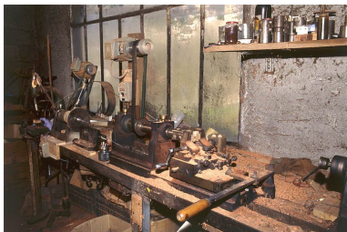
Vue d'ensemble, avec son moteur. Phot. Jérôme Mongreville IVR43_20003900993ZA
