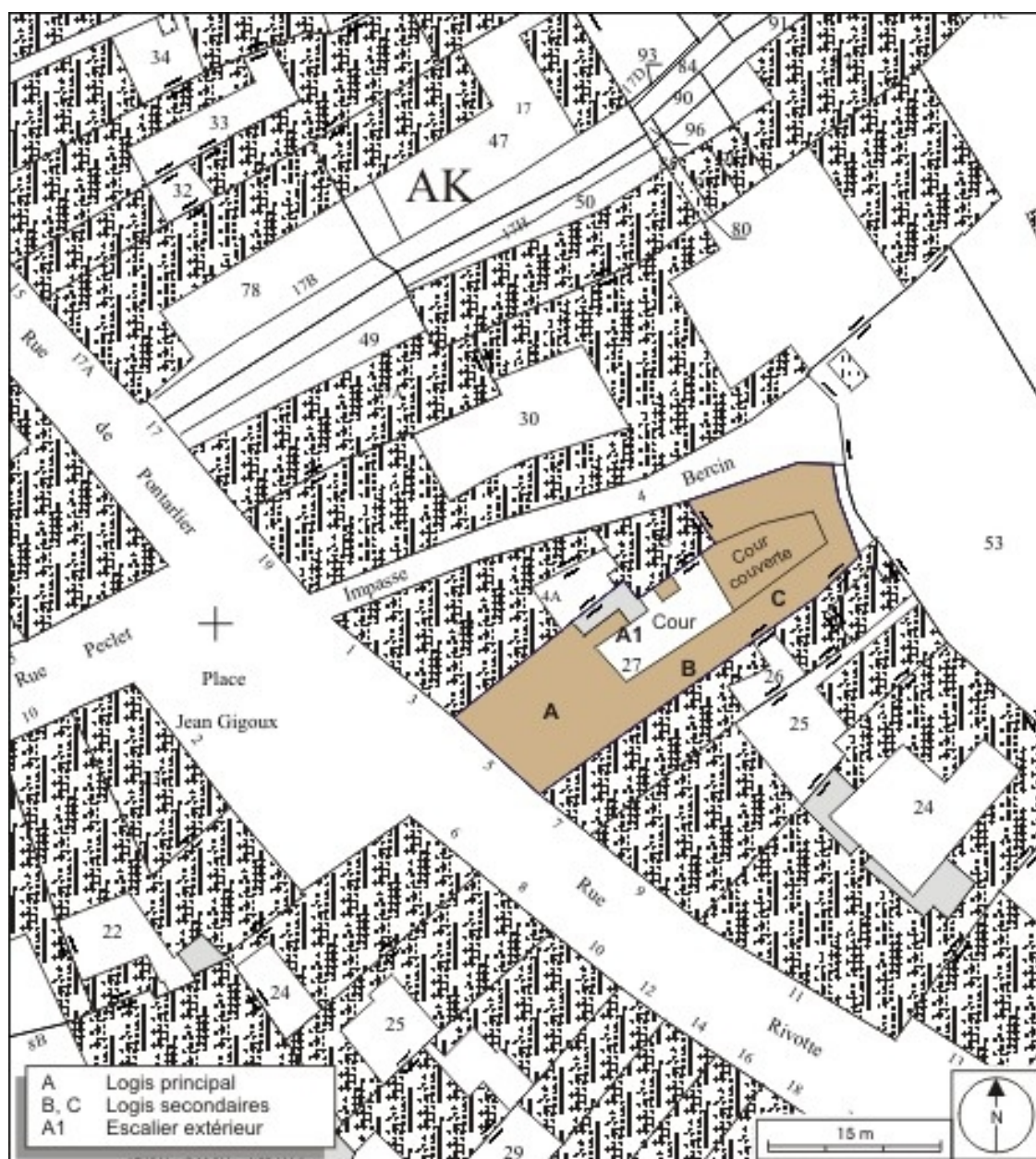
Plan masse et de situation. Extrait du plan cadastral, 1974, section AK.
