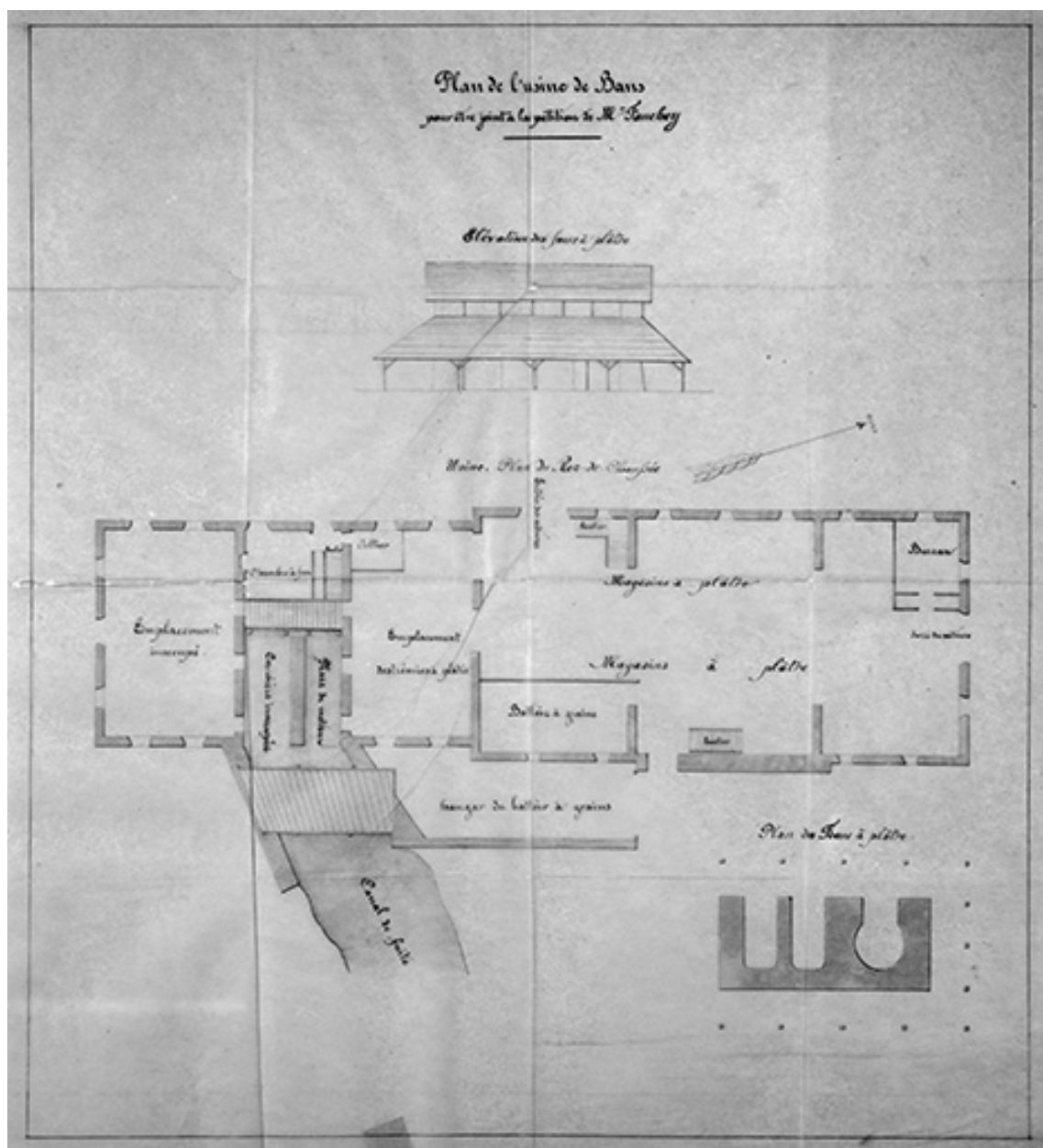
Plan de l'usine de Bans pour être joint à la pétition de M. Fauchey, plan et élévation des fours et de l'usine.
