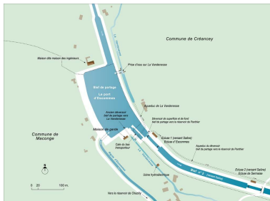
Plan schématique du port d'Escommes et du bief 02 du versant Saône. Dess. Alain Morelière IVR26_20132100094NUDA
