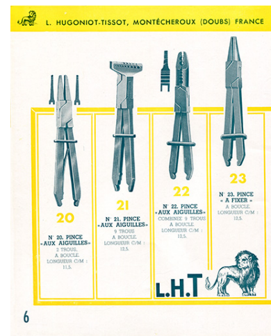
Catalogue L.H.T. 3 [catalogue de production p. 6 : pinces aux aiguilles et à fixer], [1949]. IVR43_20192500979NUC4A
