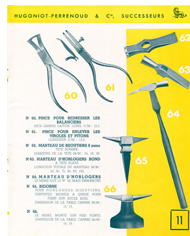
Catalogue L.H.T. 3 [catalogue de production p. 11 : pinces, marteaux et bigornes], [1949]. IVR43_20192500980NUC4A
