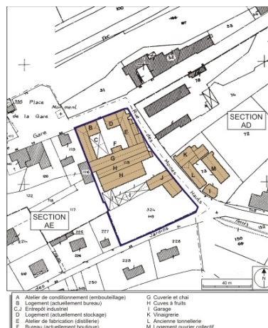
Plan-masse et de situation. Extrait du plan cadastral numérisé, 2008, section AE, 1:1000 réduit à 1:1250. Source : Direction générale des Finances Publiques - Cadastre ; mise à jour : 2008. Dess. André Céréza IVR43_20087000238NUCA
