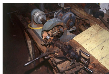
Machine à fraiser. Phot. Jérôme Mongreville IVR43_20003901061ZA
