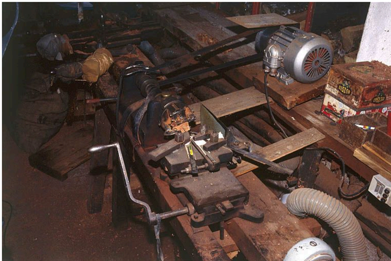
Machine à tourner dite machine à ébaucher.
