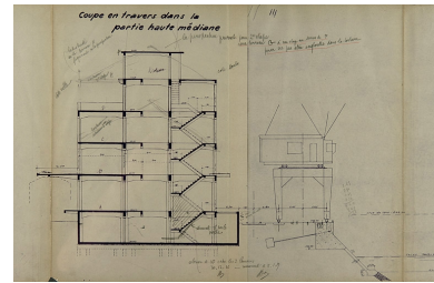
Concours pour la construction d'un entrepôt en béton armé au port de Besançon. Dessins [détail : ] Coupe en travers dans la partie haute médiane, 1936. Phot. Yves Sancey, Autr. Moreau IVR43_20062500115NUCA
