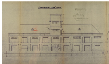
Concours pour la construction d'un entrepôt en béton armé au port de Besançon. Dessins [détail : ] Élévation côté eau, 1936. Phot. Yves Sancey, Autr. Moreau IVR43_20062500111NUCA
