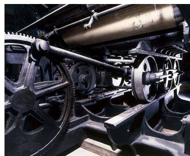
Système d'entraînement du marbre et son boggie. Le cylindre est visible en haut. Phot. Jérôme Mongreville IVR43_20013900823XA
