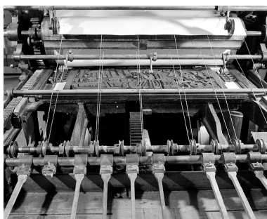
Partie arrière de la machine, vue de face. Les fils permettent de soutenir la feuille qui sera déposée sur la table de réception, à droite, à l'aide du receveur mécanique à raquettes. Phot. Jérôme Mongreville IVR43_20013900820X
