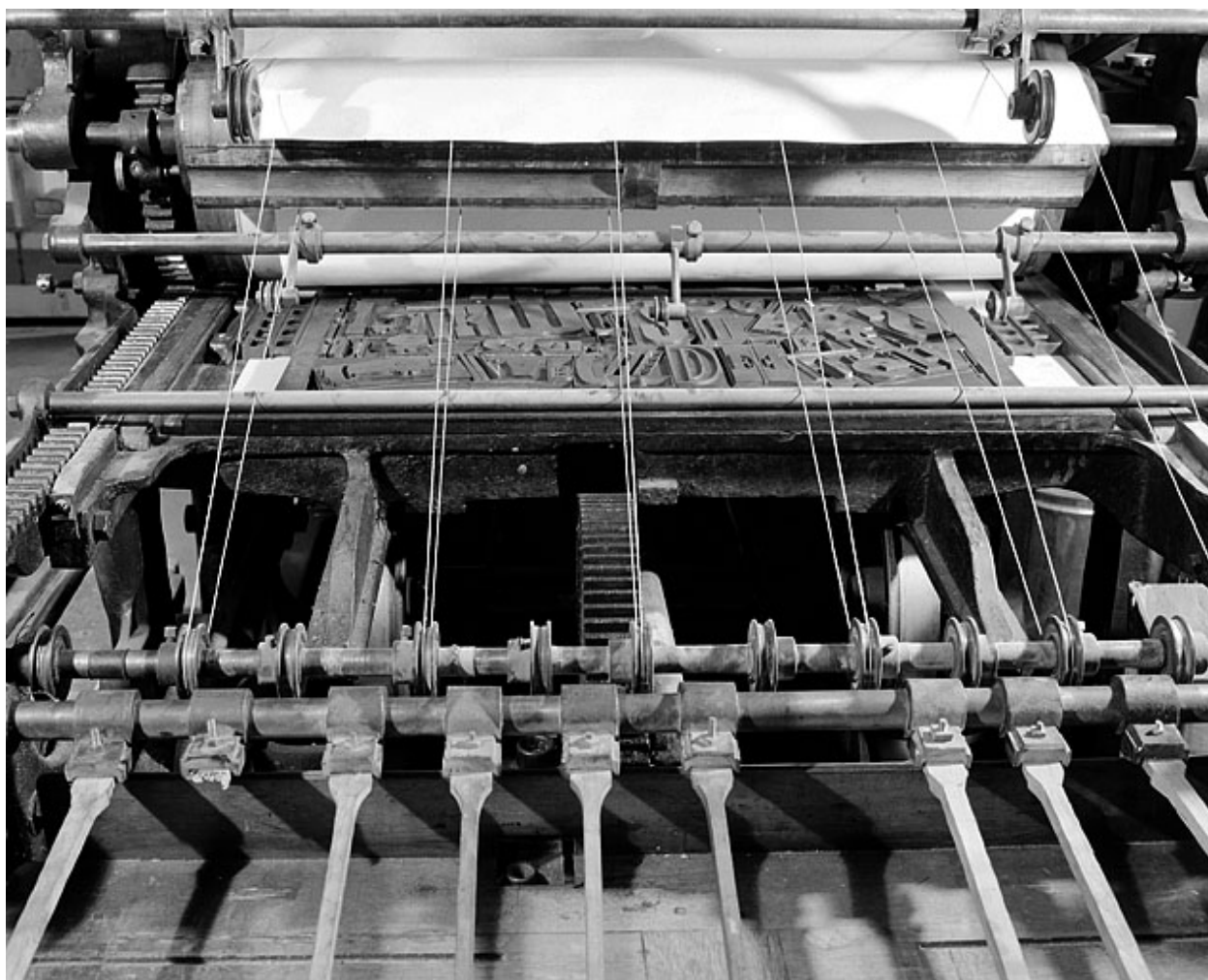
Partie arrière de la machine, vue de face. Les fils permettent de soutenir la feuille qui sera déposée sur la table de réception, à droite, à l'aide du receveur mécanique à raquettes.
