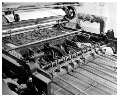
Partie arrière de la machine. Les fils permettent de soutenir la feuille qui sera déposée sur la table de réception, à droite, à l'aide du receveur mécanique à raquettes. Phot. Jérôme Mongreville IVR43_20013900821X
