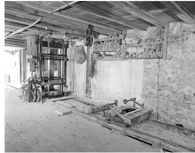
Châssis multiple et chariot. Phot. Jérôme Mongreville IVR43_19963901311X
