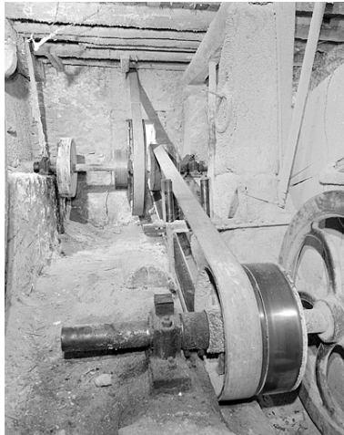
Renvoi de mouvement vers le châssis multiple. Phot. Jérôme Mongreville IVR43_19963901312X
