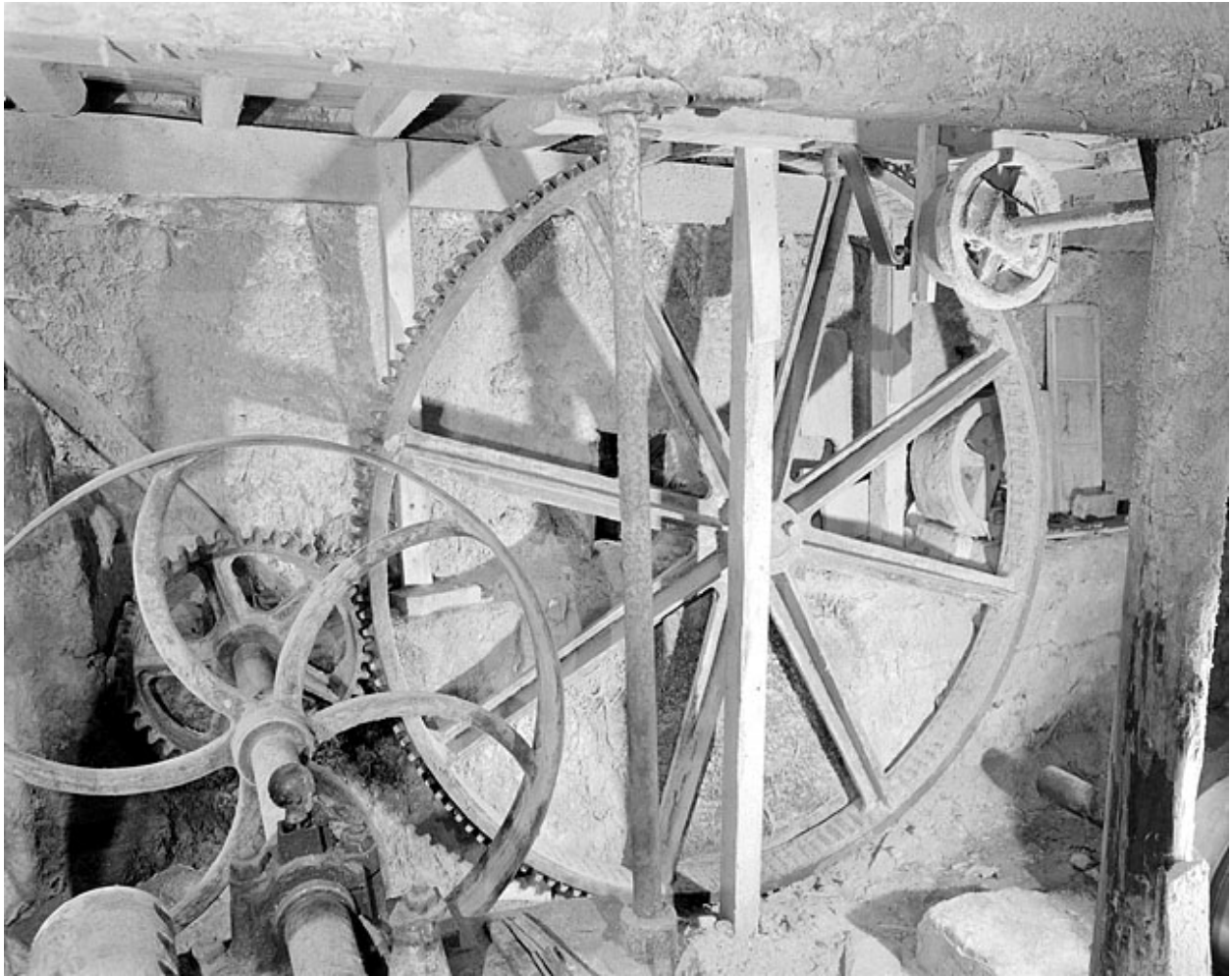
Rouet transmettant le mouvement de la roue extérieure.
