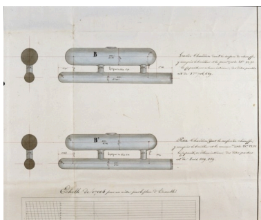
Plan du haut fourneau de Montureux appartenant à Mrs de Falatieu [les chaudières]. Phot. Yves Sancey IVR43_19907000148XA
