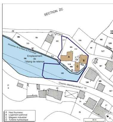
Plan-masse et de situation. Extrait du plan cadastral numérisé, 2008, section C, 1:1000. Source : Direction générale des Finances Publiques - Cadastre ; mise à jour : 2008. Dess. André Céréza IVR43_20087000991NUDA
