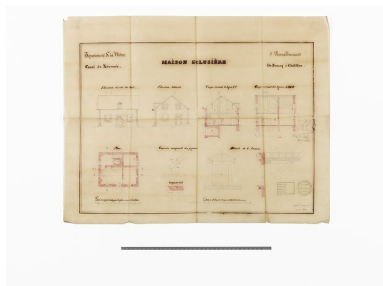
"Maison éclusière de Bernay à Châtillon". Plan, coupe et élévation et détail de la lucarne. (Archives VNF-direction territoriale Centre-Bourgogne ; subdivision de Corbigny) Phot. Thierry Kuntz IVR26_20135800011NUC4A
