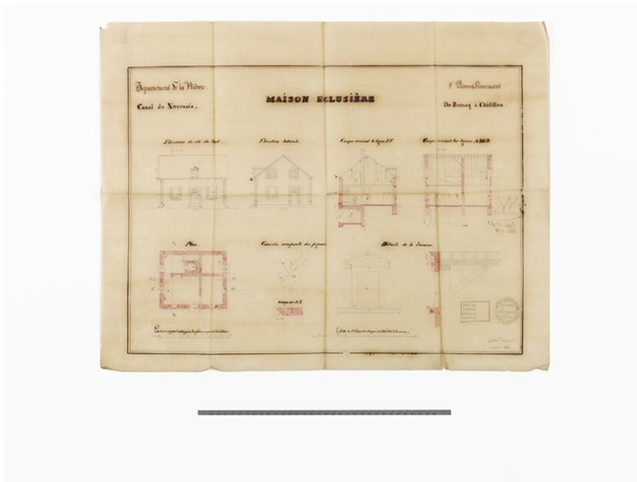
"Maison éclusière de Bernay à Châtillon". Plan, coupe et élévation et détail de la lucarne. (Archives VNF-direction territoriale Centre-Bourgogne ; subdivision de Corbigny)
