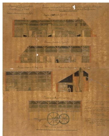
Elévation intérieure de l'usine de Sceaux-sur-Saône consistant en haut fourneau, forges et laminoir [...]. Phot. Yves Sancey, Autr. Chevillet IVR43_19877000074XA
