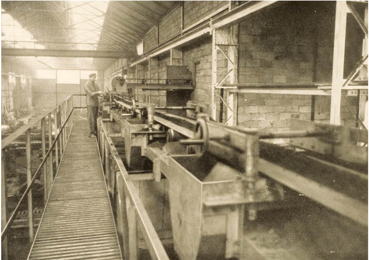
Halle de moulage. Alimentation automatique des machines à mouler.
