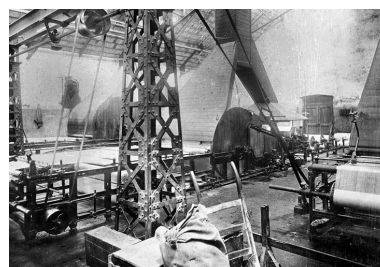
Société Anonyme de Filature et Tissage de Giromagny. Le tissage du Pont : la salle des encolleuses. Phot. Jérôme Mongreville, Autr. NEPASUTILISERDe Jongh Frères (photographe) IVR43_20019000161X
