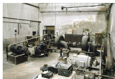
Les turbines du bâtiment d'eau. Phot. Yves Sancey IVR43_19999000286ZA
