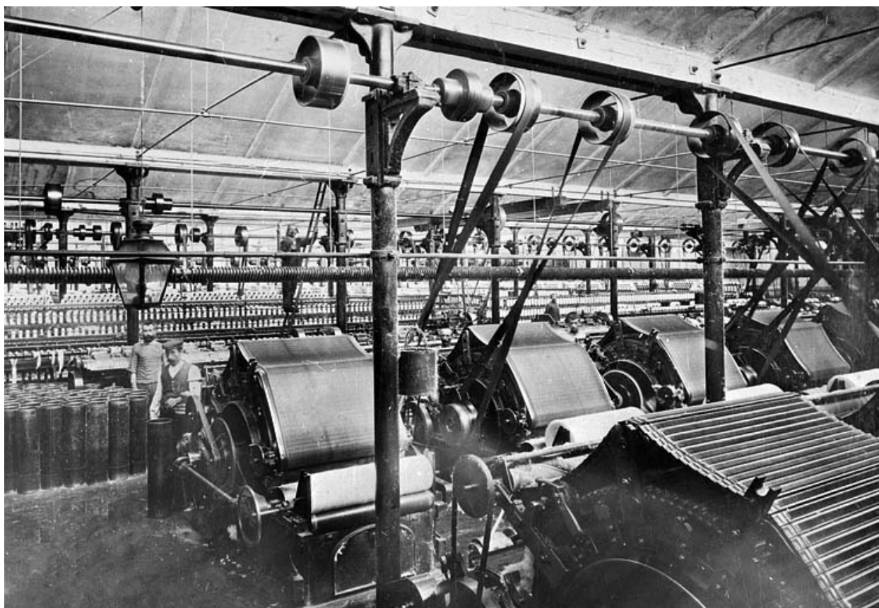
Société Anonyme de Filature et Tissage de Giromagny. Le tissage du Pont : l'atelier des caneteuses.
