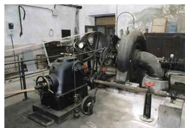
Turbine Francis (1929) et son régulateur. Phot. Yves Sancey IVR43_19999000290ZA
