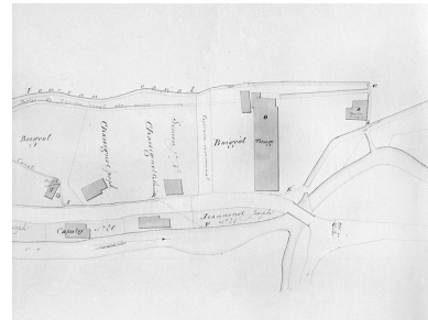
Plan à joindre au rapport [...] pour les propriétés situées le long du canal dit des Mines appartenant au sieur Boigeol et alimentant son tissage mécanique [...].
