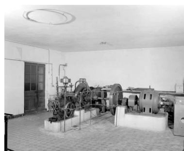
Centrale hydroélectrique : groupe ancien. Phot. Jérôme Mongreville IVR43_19923900458X
