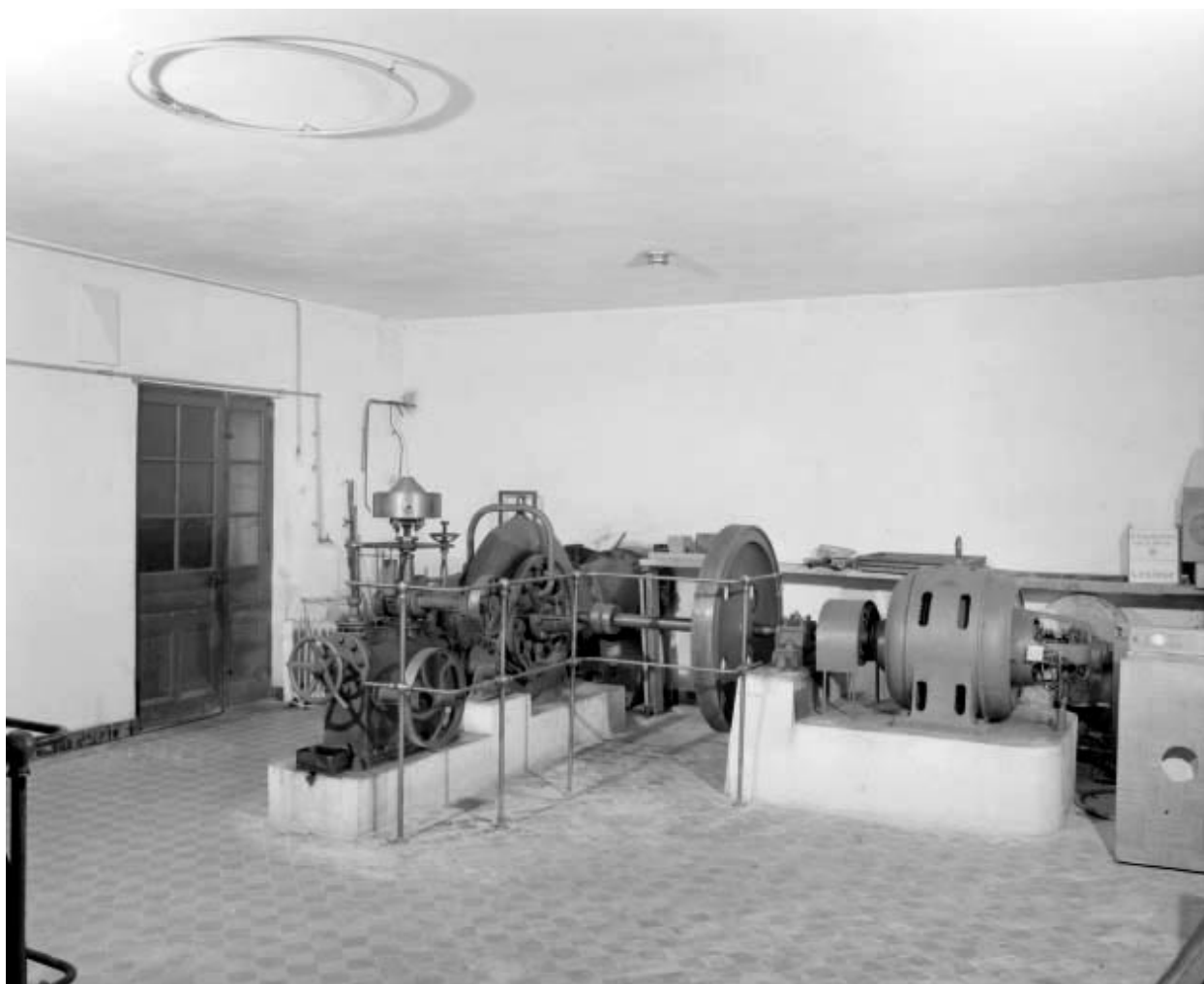
Centrale hydroélectrique : groupe ancien.
