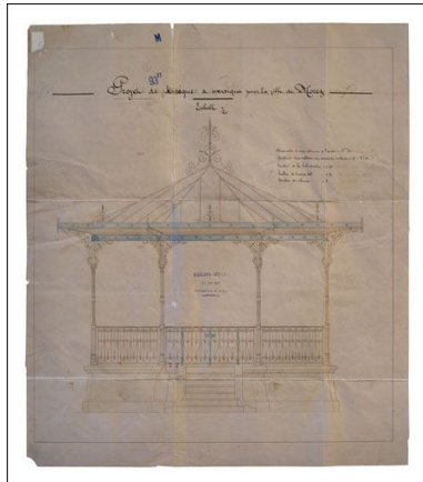
Projet de kiosque à musique pour la ville de Morez : dessin (tirage à l'ammoniaque rehaussé de lavis), 15 juin 1899, échelle 1:20. Phot. Jérôme Mongreville IVR43_20103900056NUC2A
