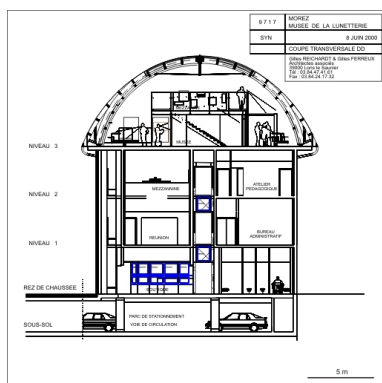
Coupe transversale DD, 2000. Dess. Gilles Reichardt, Dess. Gilles Ferreux, IVR43_20103900151NUDA
