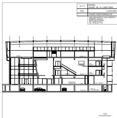
Coupe longitudinale AA, 2000. Dess. Gilles Reichardt, Dess. Gilles Ferreux, IVR43_20103900147NUDA
