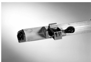
Blocage de l'équerre de l'un des composteurs métalliques : système à levier à axe vertical. Phot. Jérôme Mongreville IVR43_20023900083X
