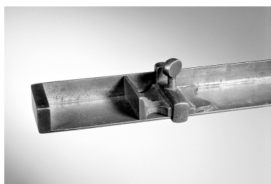
Blocage de l'équerre de l'un des composteurs métalliques : système à vis. Phot. Jérôme Mongreville IVR43_20023900079X
