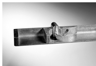
Blocage de l'équerre de l'un des composteurs métalliques : système à levier à axe horizontal. Phot. Jérôme Mongreville IVR43_20023900080X
