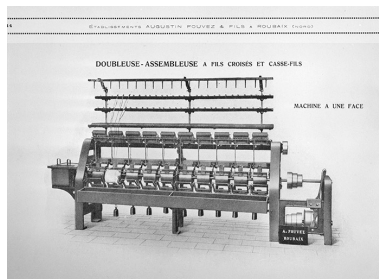
Doubleuse-assembleuse à fils croisés et casse-fils. Phot. Yves Sancey IVR43_19953900117X
