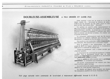
Doubleuse-assembleuse à fils croisés et casse-fils. Phot. Yves Sancey IVR43_19953900114X
