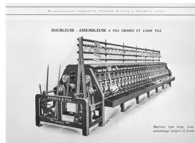
Doubleuse-assembleuse à fils croisés et casse-fils. Phot. Yves Sancey IVR43_19953900118X
