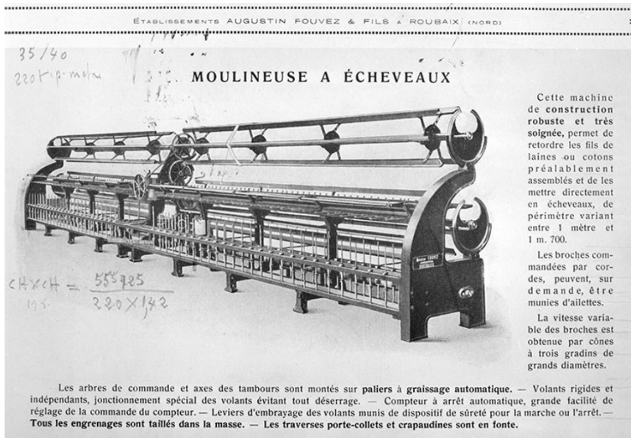
Moulineuse à écheveaux.
