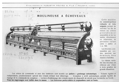
Moulineuse à écheveaux. Phot. Yves Sancey IVR43_19953900113X
