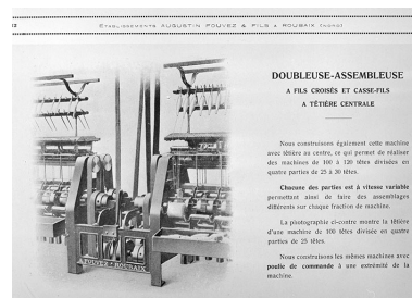
Doubleuse-assembleuse à fils croisés et casse-fils à têtère centrale. Phot. Yves Sancey IVR43_19953900115X
