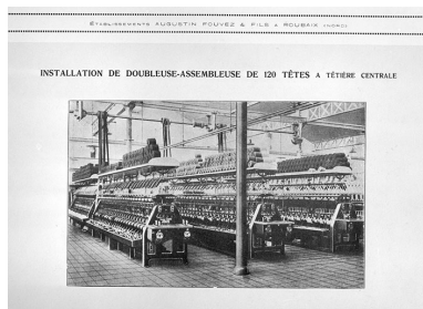
Installation de doubleuse-assembleuse de 120 têtes à têtère centrale. Phot. Yves Sancey IVR43_19953900116X
