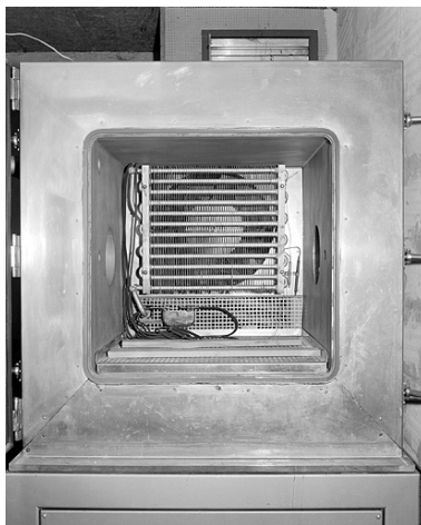
Enceinte d'essais : intérieur. Phot. Jérôme Mongreville IVR43_20032501036X
