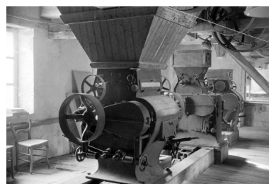
Minoterie, étage : les appareils à cylindres. Phot. Laurent Poupard IVR43_19883900646Z
