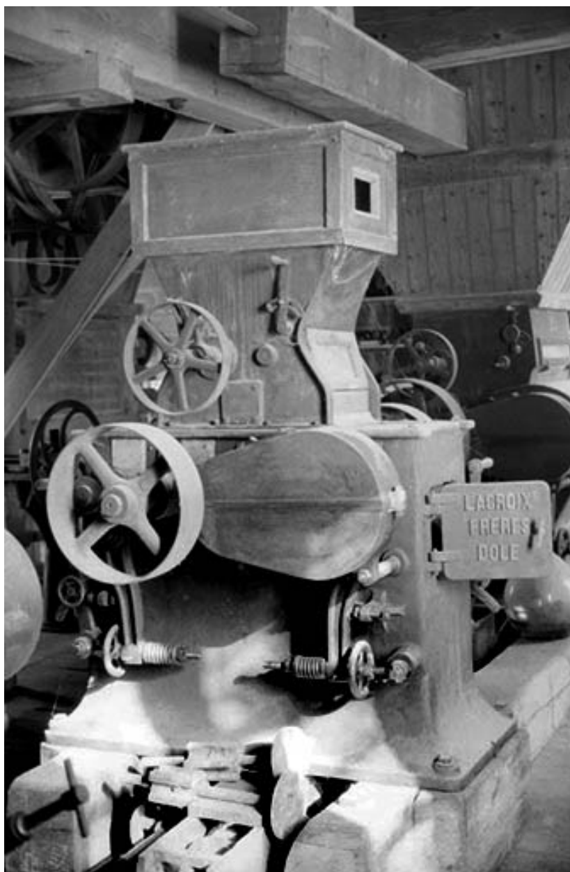
Minoterie, étage : appareil à cylindres Lacroix.
