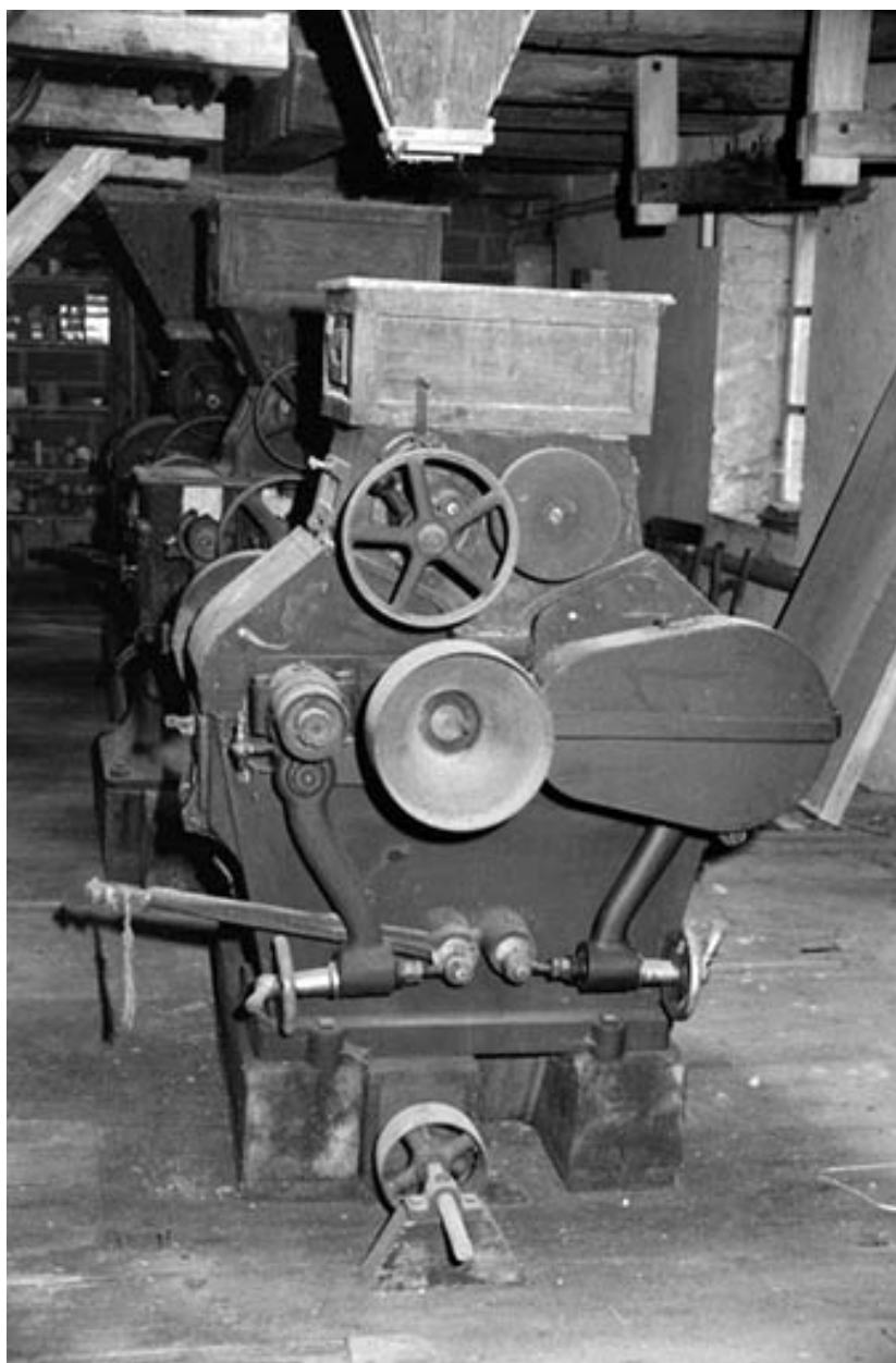
Minoterie, étage : appareil à cylindres.
