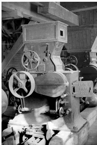
Minoterie, étage : appareil à cylindres Lacroix. Phot. Laurent Poupard IVR43_19883900647Z
