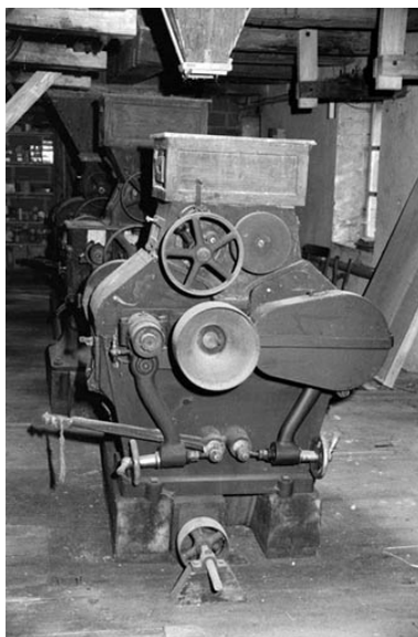
Minoterie, étage : appareil à cylindres. Phot. Laurent Poupard IVR43_19883900648Z
