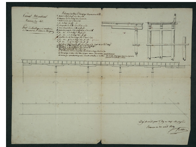
Pont de halage à construire à l'amont de l'écluse de Tarragnoz, 1829. Phot. Yves Sancey, Phot. Rance IVR43_20062500054NUCA
