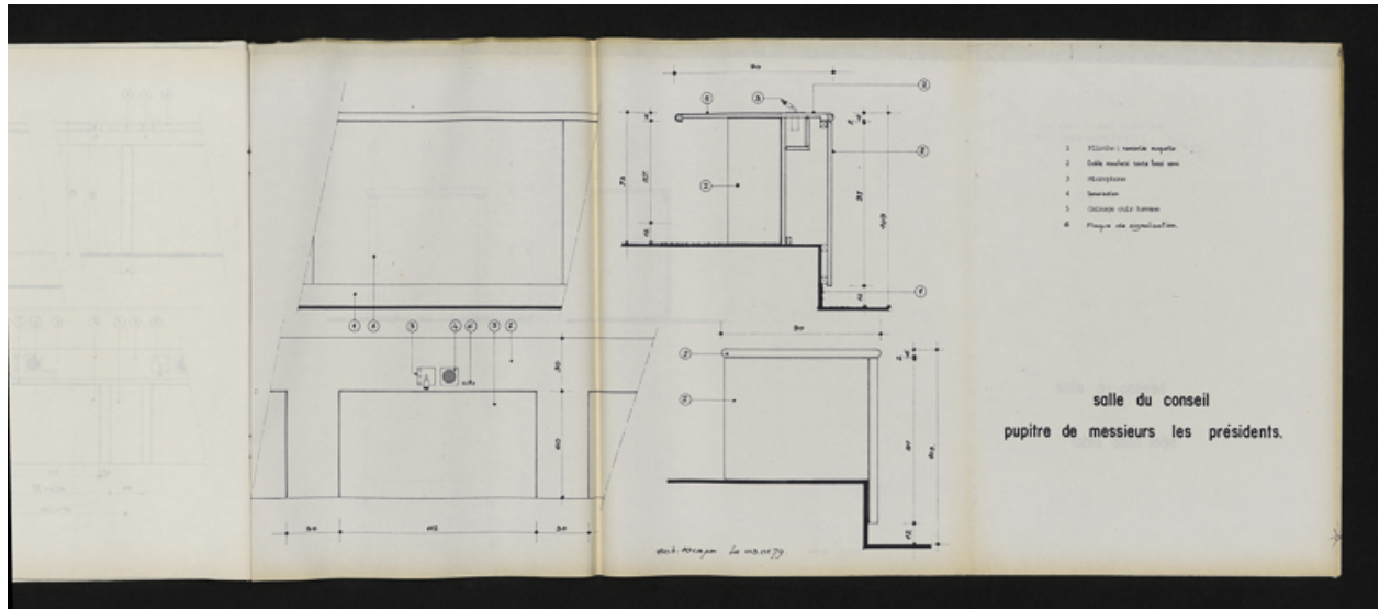
Carnet de détails et principes - salle du conseil : pupitre des présidents, plan, coupe, élévations, 3 janvier 1979. Boyer, Michel (architecte d'intérieur) (Archives départementales de la Côte-d'Or, Dijon, 32 J 106)
