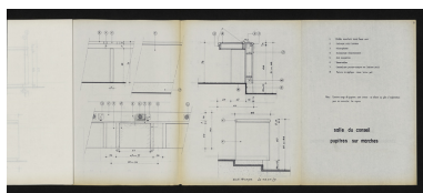
Carnet de détails et principes - salle du conseil : pupitres sur marche, 3 janvier 1979. Boyer, Michel (architecte d'intérieur)
