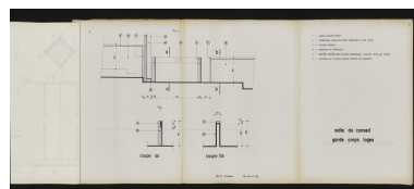
Carnet de détails et principes - salle du conseil : garde-corps des loges, 3 janvier 1979. Boyer, Michel (architecte d'intérieur)
