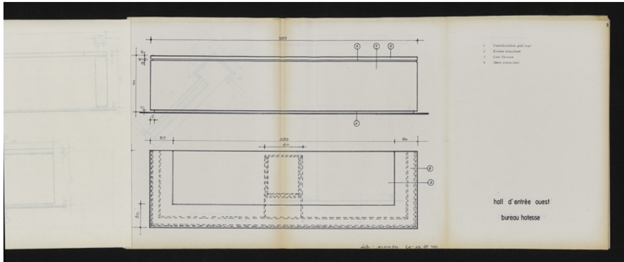
Carnet de détails et principes - hall d'entrée ouest : bureau des hôteses, plan et élévation, 13 novembre 1978. Boyer, Michel (architecte d'intérieur) (Archives départementales de la Côte-d'Or, Dijon, 32 J 106)
