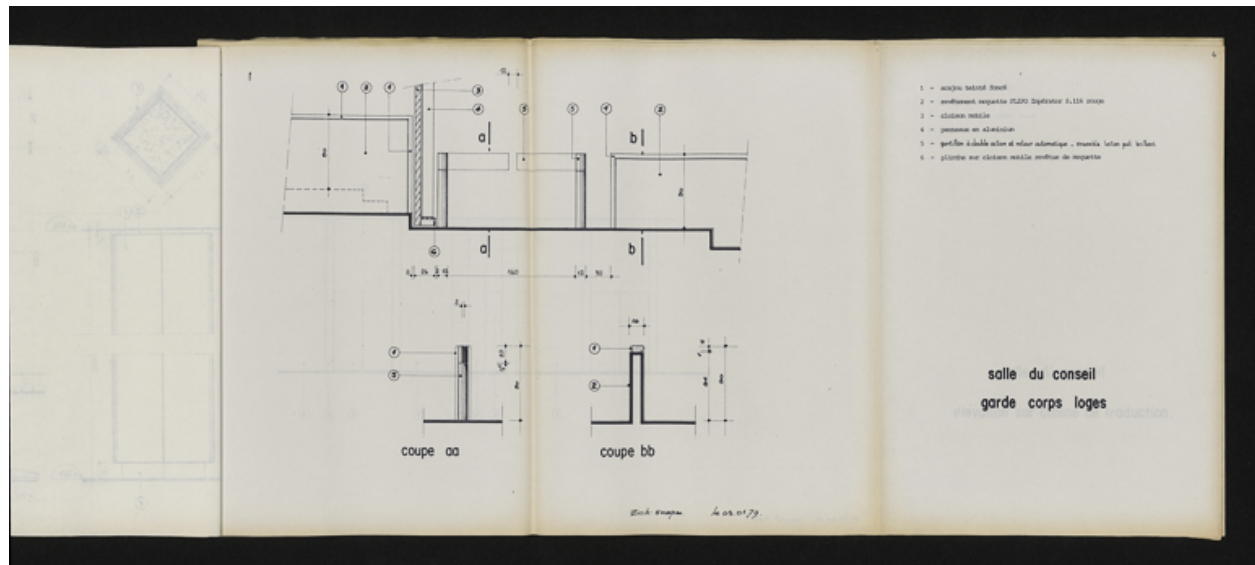
Carnet de détails et principes - salle du conseil : garde-corps des loges, 3 janvier 1979. Boyer, Michel (architecte d'intérieur) (Archives départementales de la Côte-d'Or, Dijon, 32 J 106)
