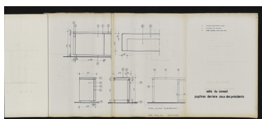
Carnet de détails et principes - salle du conseil : deuxième rangée de pupitres de la tribune, plan, coupe et élévations, 6 novembre 1978. (Archives départementales de la Côte-d'Or, Dijon, 32 J 106) Phot. Petot Frédéric IVR26_20142100777NUC2A
