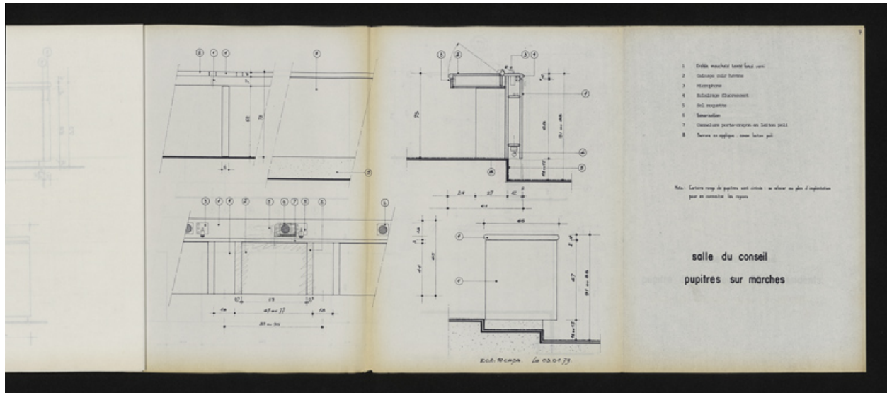
Carnet de détails et principes - salle du conseil : pupitres sur marche, 3 janvier 1979. Boyer, Michel (architecte d'intérieur) (Archives départementales de la Côte-d'Or, Dijon, 32 J 106)
