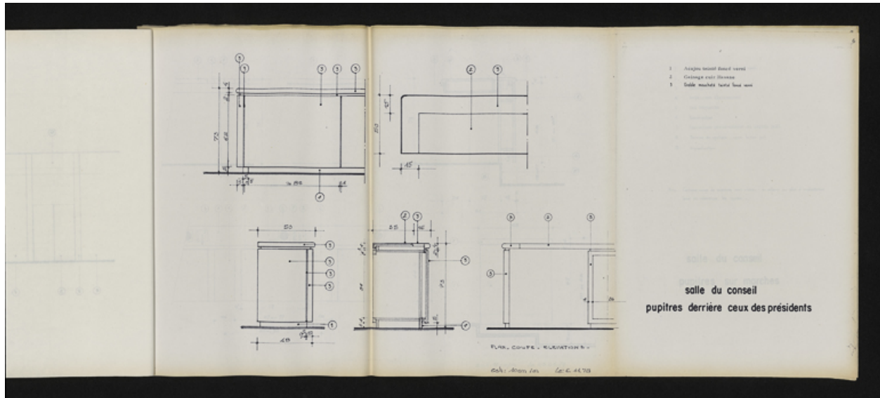
Carnet de détails et principes - salle du conseil : deuxième rangée de pupitres de la tribune, plan, coupe et élévations, 6 novembre 1978. (Archives départementales de la Côte-d'Or, Dijon, 32 J 106)
