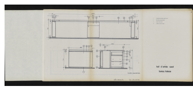
Carnet de détails et principes - hall d'entrée ouest : bureau des hôtes, coupe et élévations, 13 novembre 1978. Boyer, Michel (architecte d'intérieur) (Archives départementales de la Côte-d'Or, Dijon, 32 J 106) Phot. Petot Frédéric, Autr. Michel (architecte d'intérieur) Boyer IVR26_20142100796NUC2A
