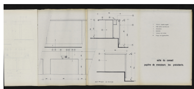
Carnet de détails et principes - salle du conseil : pupitre des présidents, plan, coupe, élévations, 3 janvier 1979. Boyer, Michel (architecte d'intérieur)
