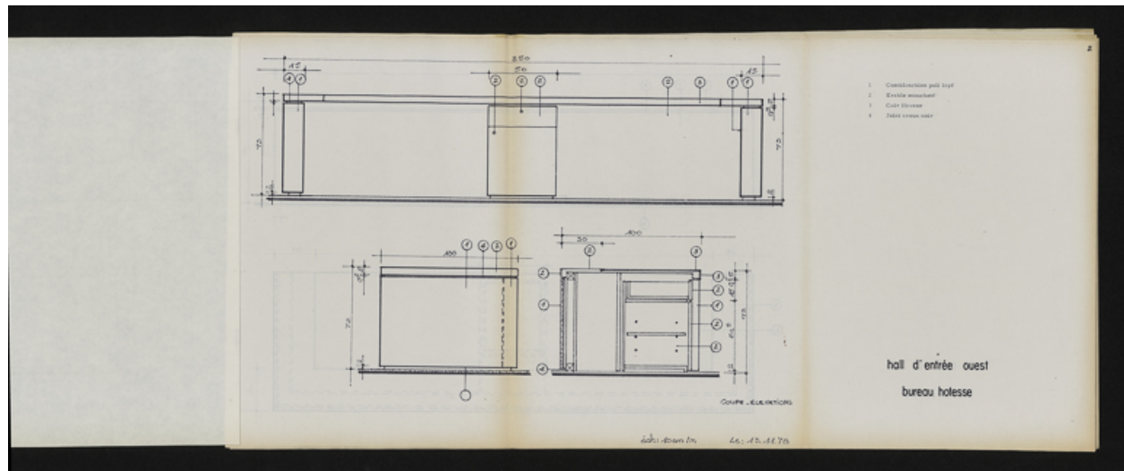
Carnet de détails et principes - hall d'entrée ouest : bureau des hôtes, coupe et élévations, 13 novembre 1978. Boyer, Michel (architecte d'intérieur) (Archives départementales de la Côte-d'Or, Dijon, 32 J 106)
