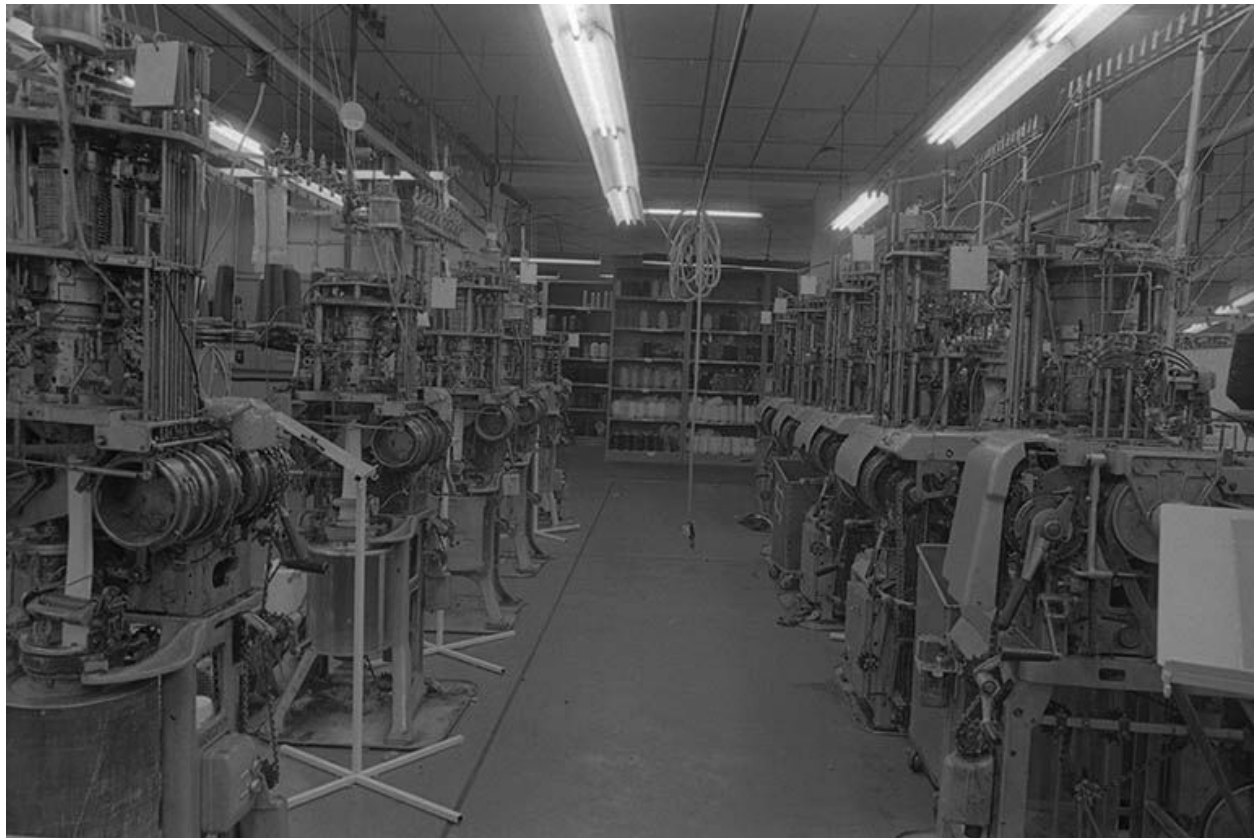
Atelier de tricotage (machines des années 1950) : vue générale.
