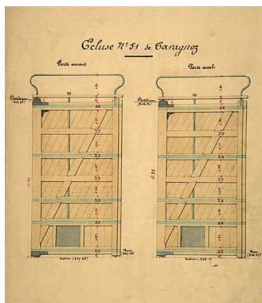
Dessin des portes de l'écluse n° 51 à placer lors de son allongement et de son exhaussement, 1879. Phot. Yves Sancey, Phot. Paul Schoendoerffer IVR43_20062500106NUCA
