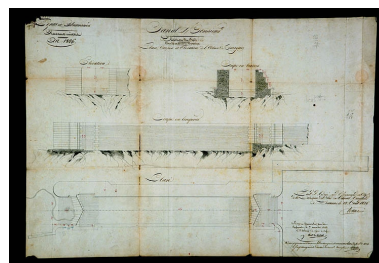
Plan, coupes et élévation de l'écluse de Taragnoz, 1826. Phot. Yves Sancey, Phot. Rance IVR43_20062500046NUCA
