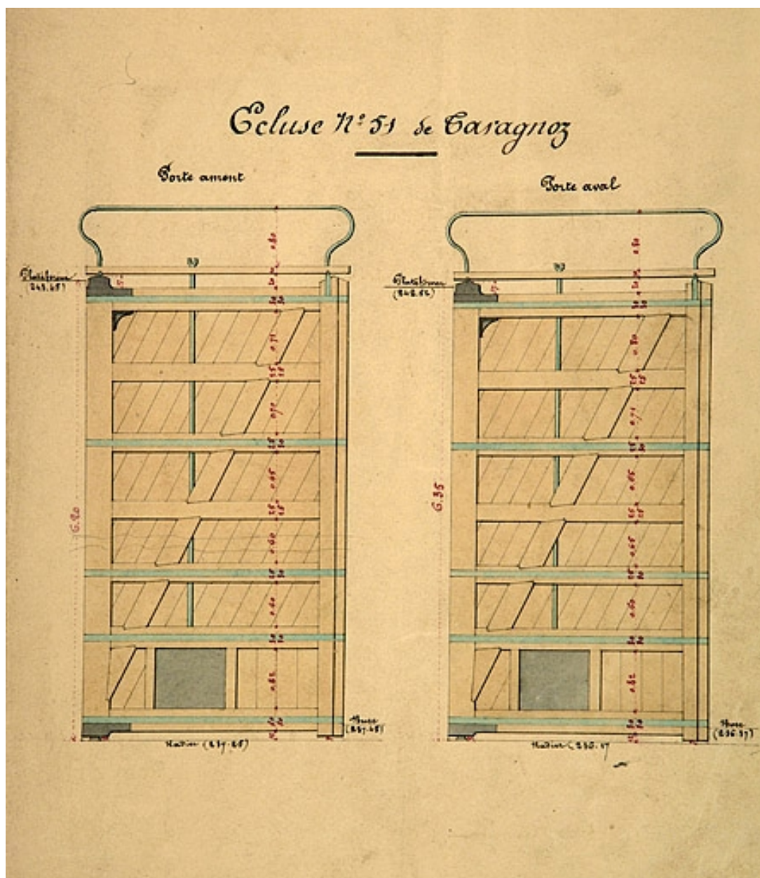
Dessin des portes de l'écluse n° 51 à placer lors de son allongement et de son exhaussement, 1879.
