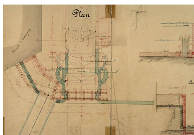
Dérivation sous la citadelle de Besançon. Dessins de détails de l'allongement par l'amont de l'écluse n° 51 [plan et coupes], 1877. Phot. Yves Sancey, Phot. Rascol IVR43_20062500107NUCA
