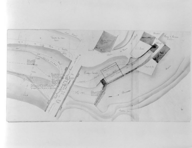
Demande de construction d'un barrage des Srs Lamy et Lacroix. Plan général [détail de la partie droite]. Dessin, 1859. Echelle 1:200.
