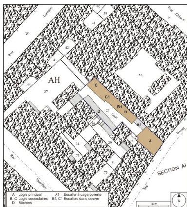
Plan masse et de situation. Extrait du plan cadastral, 1974, section AH. Dess. André Céréza IVR43_20102500072NUDA
