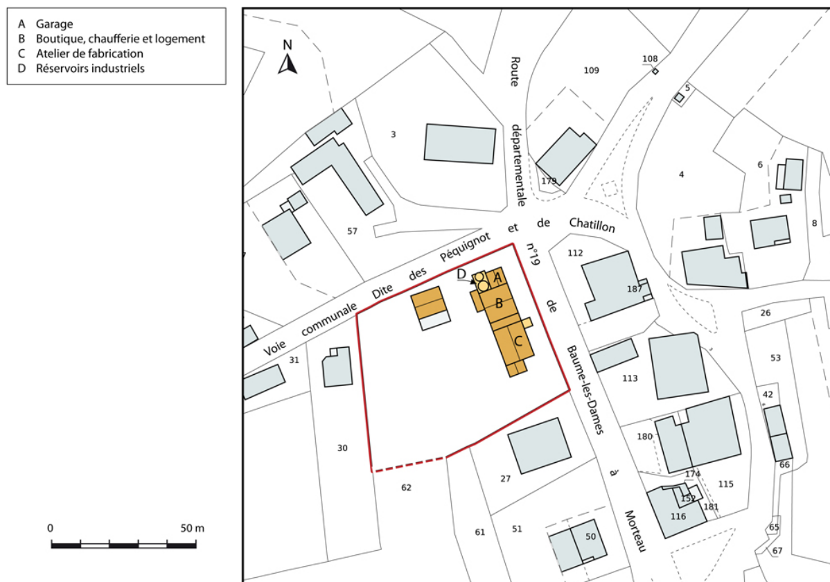
Plan-masse et de situation. Extrait du plan cadastral, 2014, section ZC.
