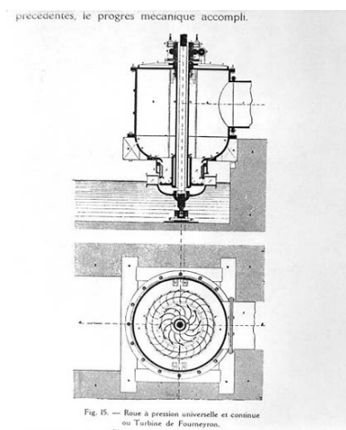
Détail du dessin et de la coupe de la turbine Fourneyron (1832). Phot. Yves Sancey, Autr. Benoît Fourneyron IVR43_19933900546X
