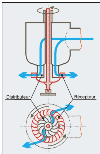
Schéma de principe de la turbine Fourneyron. D'après un dessin et une coupe publiés dans : " Cent ans de mécanique : Centenaire des ateliers Crozet-Fourneyron 1832-1932 ", Paris : Poyet, 1932, p. 14. Dess. André Céréza IVR43_20013900827NUDA
